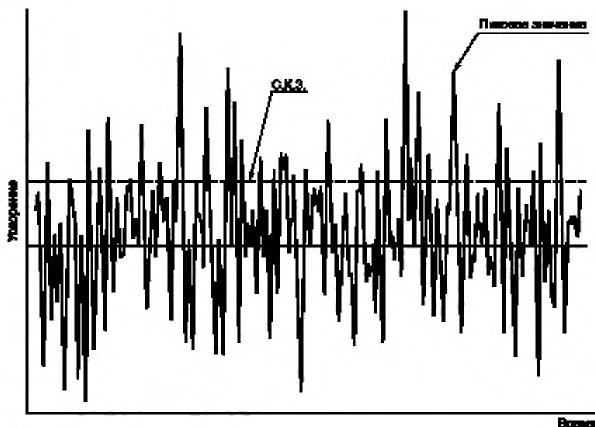
Рисунок A.2 — Отсечка (ограничение) сигнала
