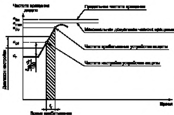
Рисунок 1 — Типичная кривая срабатывания устройства защиты
