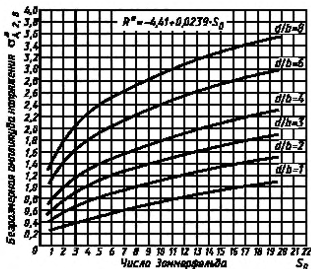
Рисунок А.3 — Антифрикционный слой/промежуточный слой:
