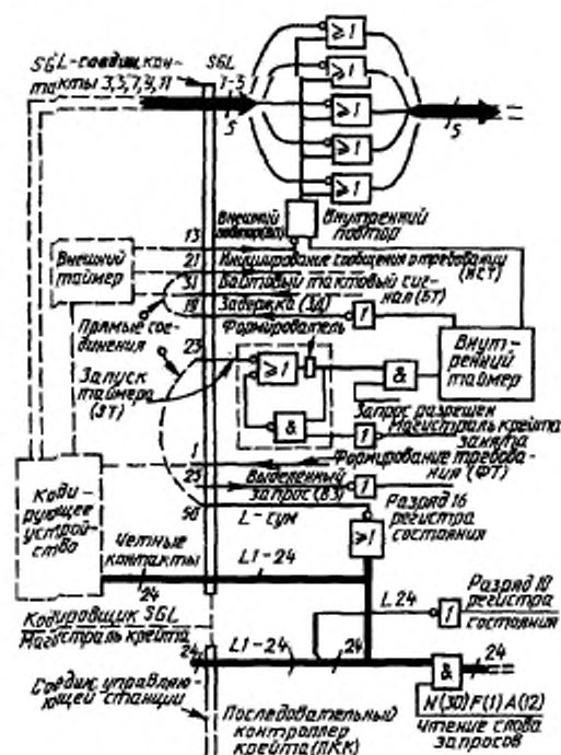
Пример схемы взаимодействия ПКК и кодировщика
