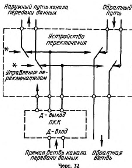
Пример переключения схемы для одного сигнала D-порта
