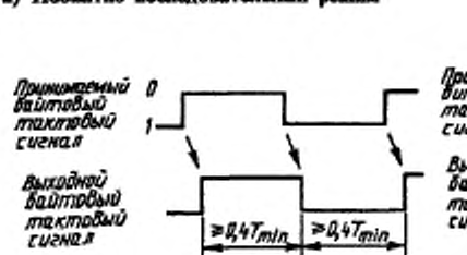
Соотношения между байтовыми тактовыми сигналами на соединителе и принимаемыми битовыми/байтовыми тактовыми сигналами
