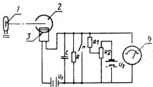
1 — нормированный источник света; 2 — светоприемный блок; 3 — светоприемник; U_1 , U_2 — источники тока; C — интегрирующий конденсатор; R — резистор для калибровки; n — замыкающий переключатель; R_1 , R_2 — резисторы для компенсации темного тока; 4 — вольтметр
