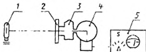
1 — нормированный источник света, 2 — линзовое стекло, 3 — испытуемый фотоаппарат, 4 — блок оптического блока, 5 — контрольно-измерительный прибор.
