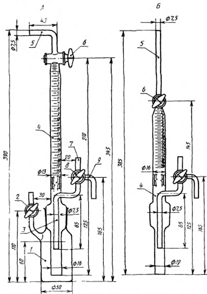
1 — склянка со шлифом; 2 — кран; 3, 7, 9 — отростки крана; 4 — бюретка со шлифом (А — цена деления — 0,1 см 3 , Б — цена деления — 0,2 см 3 ); 5 — отросток бюретки; 6 — кран бюретки; 8 — трехходовой кран
