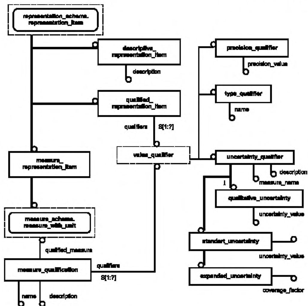
Рисунок D.3 — qualified_measure_schema —EXPRESS-G диаграмма 1 из 1
