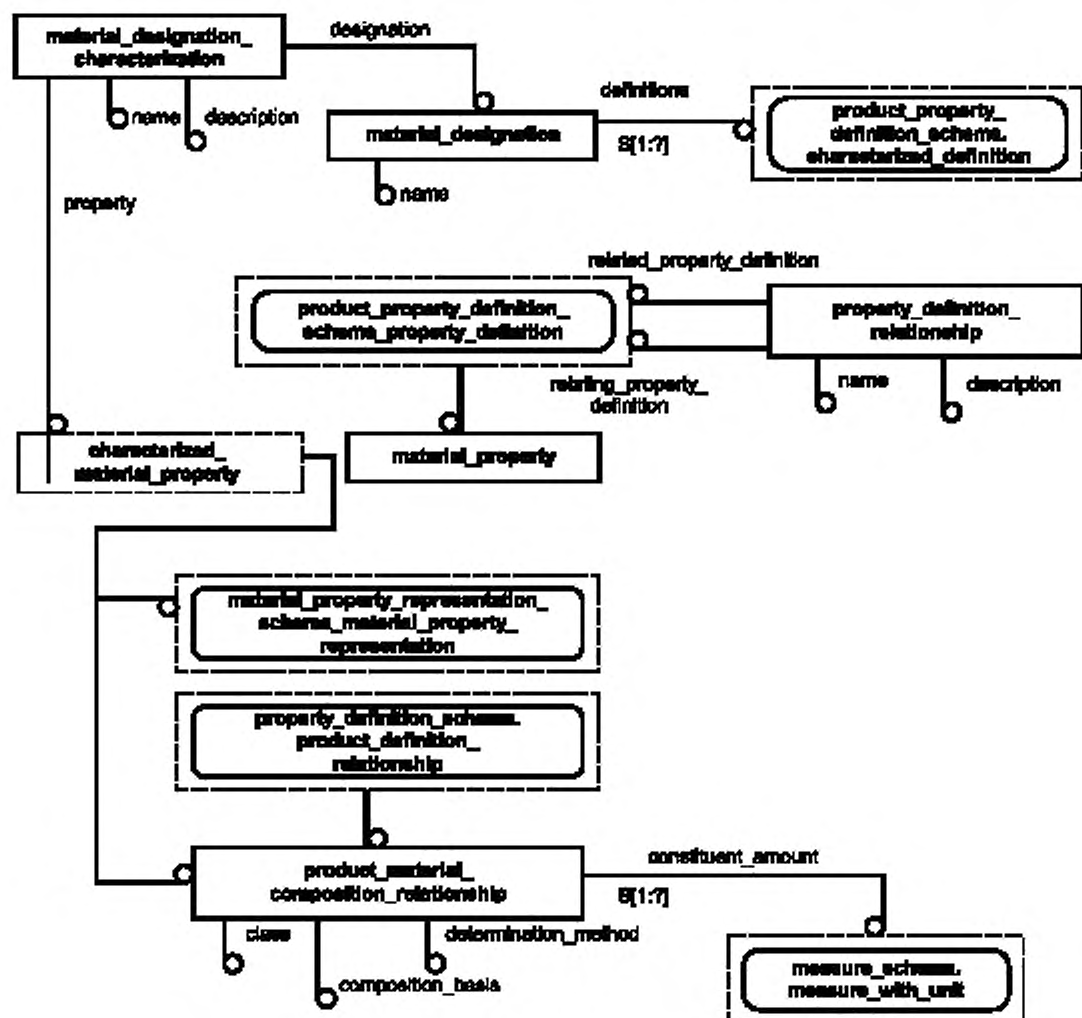
Рисунок D.1 — material_property_definition_schema — EXPRESS-G диаграмма 1 из 1
