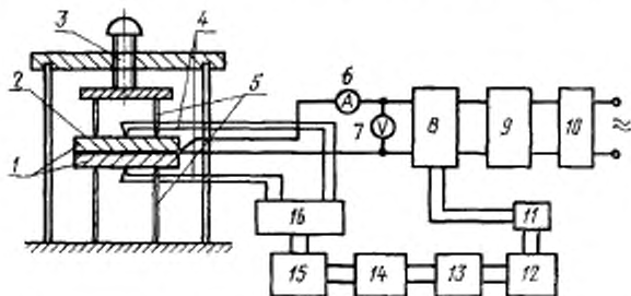
1—исследуемый образец; 2—нагреватель; 3—прижимной винт; 4—термометр; 5—иглочатые держатели; 6—миллиамперметр; 7—вольтметр; 8—электромагнитное реле; 9—генератор; 10—выпрямитель; 11—реле; 12—самовоссец электронный; 13—усилитель; 14—магазин сопротивлений; 15—потенциометр; 16—переключатель
