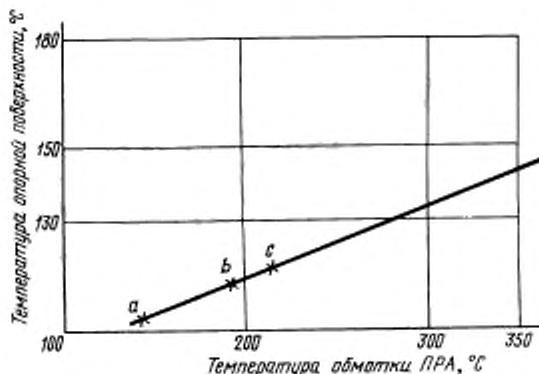
а, б, с — измеренные значения температуры при 0,9-, 1,0 и 1,1-кратном номинального напряжения
