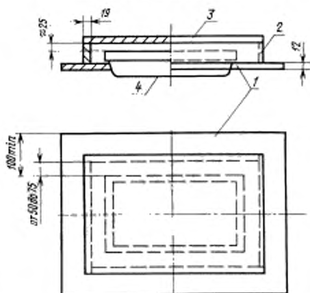
1 — основа, 2 — боковая стенка, 3 — верхняя стенка, 4 — встраиваемый светильник
