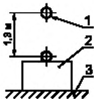
1 — стальной шарик; 2 — светильник; 3 — опорная поверхность Черт. 7а
