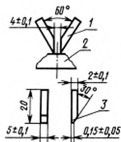
1 — электрод; 2 — испытуемый образец; 3 — конец электрода скрутки Черт. 4
