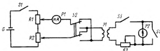
M — катушка взаимной индуктивности; R_3 — магазин сопротивлений для обеспечения режима успокоения гальванометра
