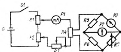
R_5 , R_6 , R_7 — сопротивления плеч измерительного моста постоянного тока; P_2 — нулевой указатель измерительного моста; P_3 — поверяемый гальванометр
