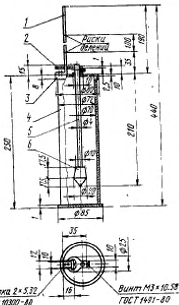
1—шкала; 2—ограничитель; 3—крышка; 4—цилиндр; 5—стержень; 6—груз.
