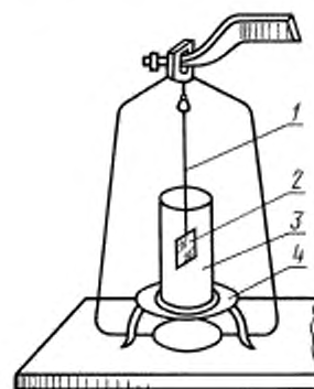
1 — проволока; 2 — образец; 3 — стакан; 4 — подставка
