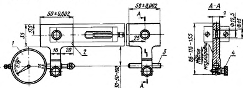
1 — индикатор; 2 — боковик; 3 — регулируемая пятка; 4 — зажимной винт.
