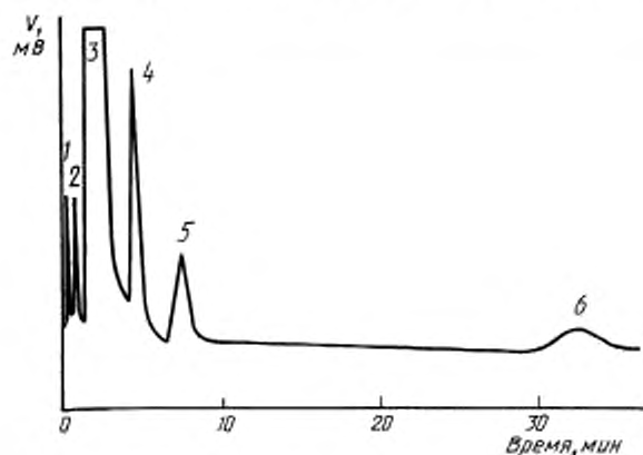
Типовая хроматограмма этиленгликоля с использованием колонки II
