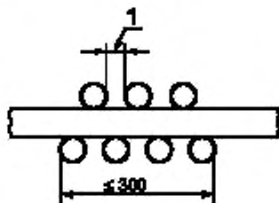
1 — зазор
