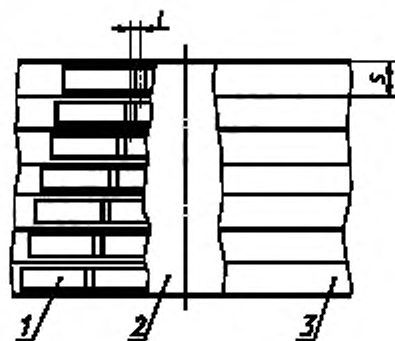
1 — образец; 2 — наплавленный валик; 3 — брусок
