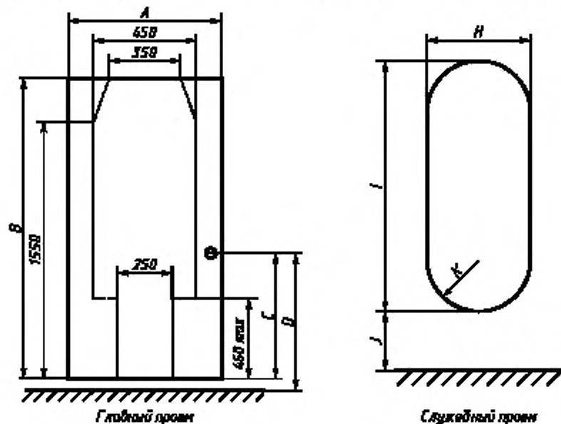
Рисунок 4 — Проемы кабин
