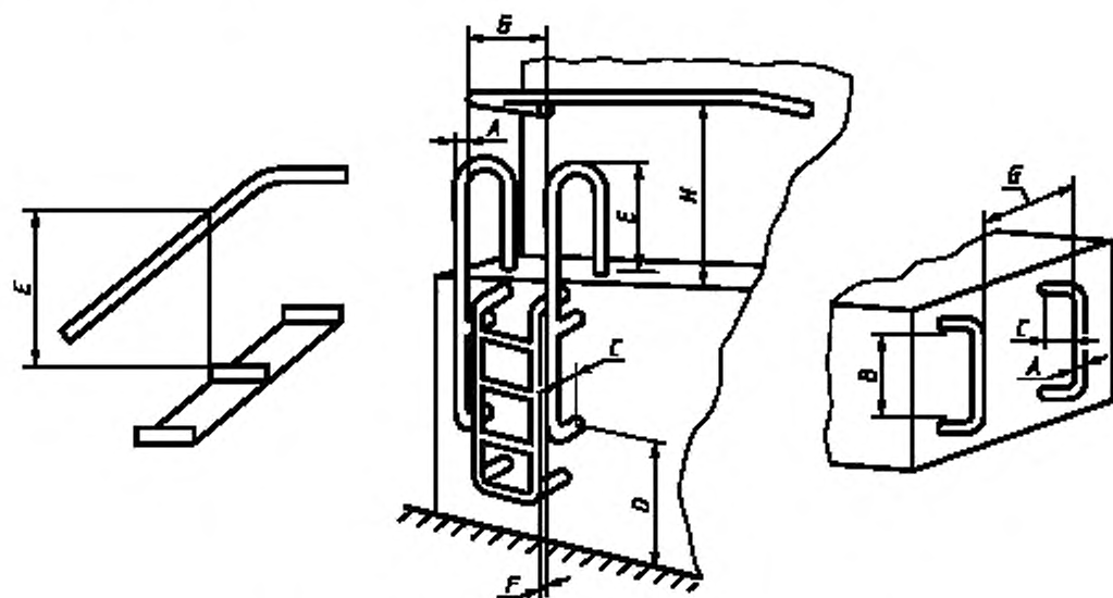
Рисунок 2 — Поручни и скобы
