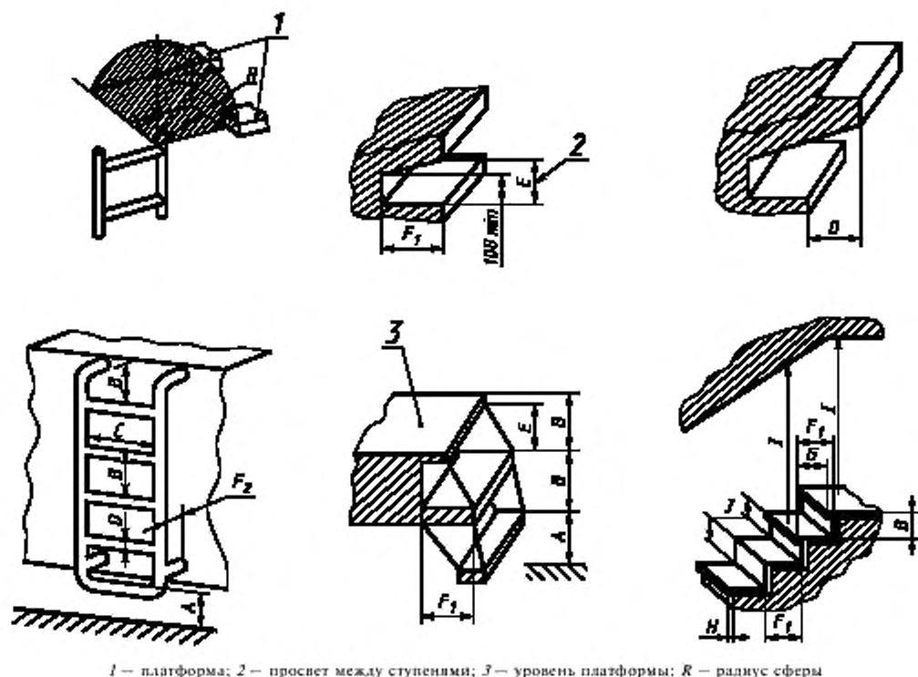
Рисунок 1 — Лестницы, трапы, ступени, перекладины
