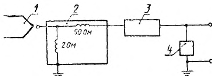
1 — ИГ; 2 — мишень; 3 — аттенюатор; 4 — осциллограф
