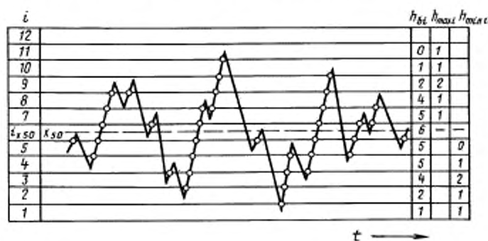
Распределения, полученные по методу пересечений
