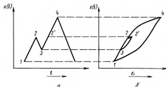
а — фрагмент процесса нагружения; б — диаграмма «напряжение — деформация»
