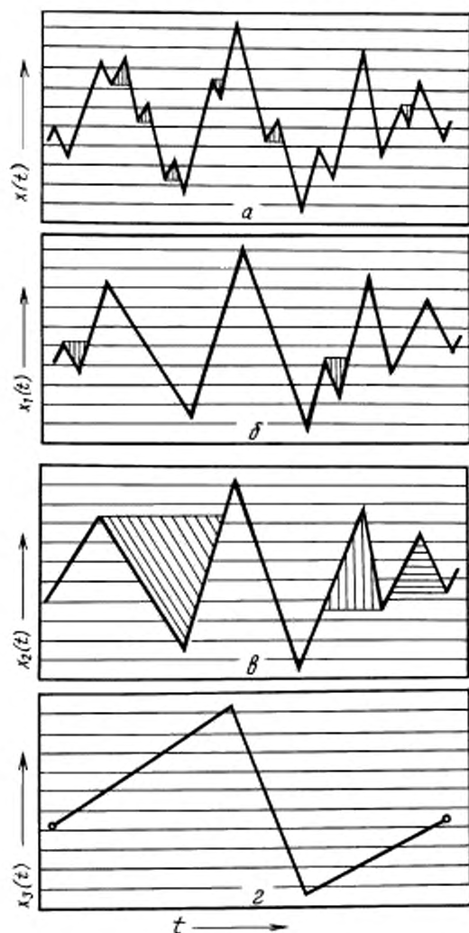
Схематизация по методу полных циклов
