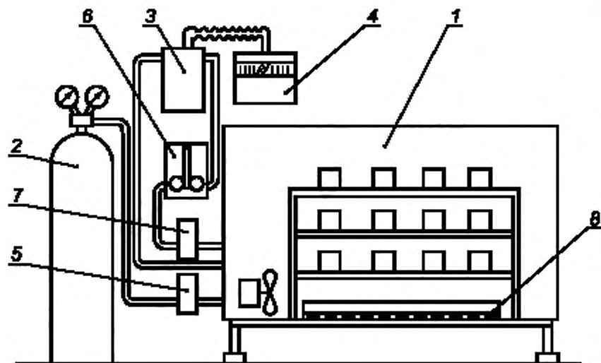
1 — камера; 2 — баллон с \text{CO}_2 ; 3 — автоматический газоанализатор; 4 — показывающий командный прибор; 5 — электромагнитный клапан; 6 — блок регулирования; 7 — лобудитель расхода газа, 8 — ванна с раствором хлорида натрия
