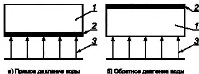
1 — испытываемый образец; 2 — защитное покрытие; 3 — направление подачи воды
