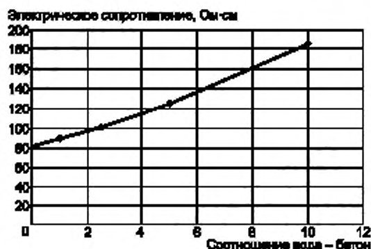
Рисунок 4 — Оценка электрического сопротивления водной вытяжки из бетона
