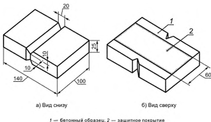
Рисунок 7 — Общий вид образца для определения трещиностойкости
