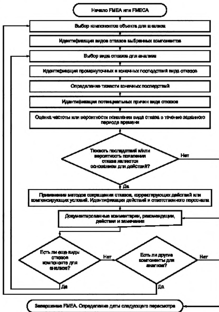
Рисунок 2 — Блок-схема анализа
