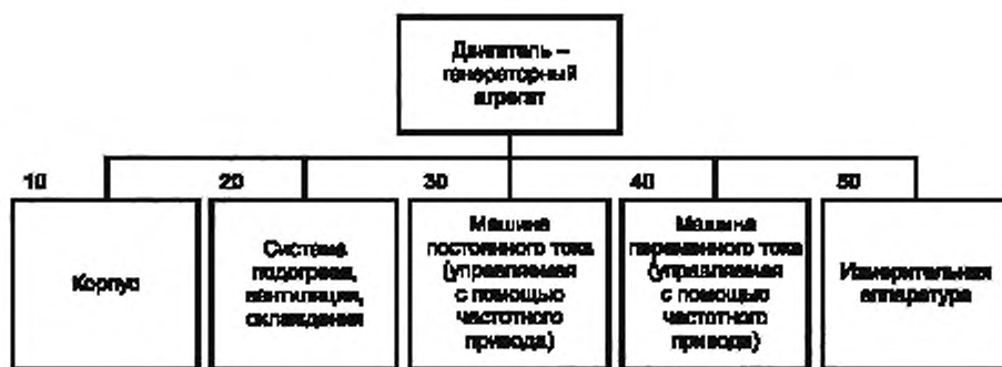
Рисунок В.2 — Диаграмма подсистем двигателя—генератора
