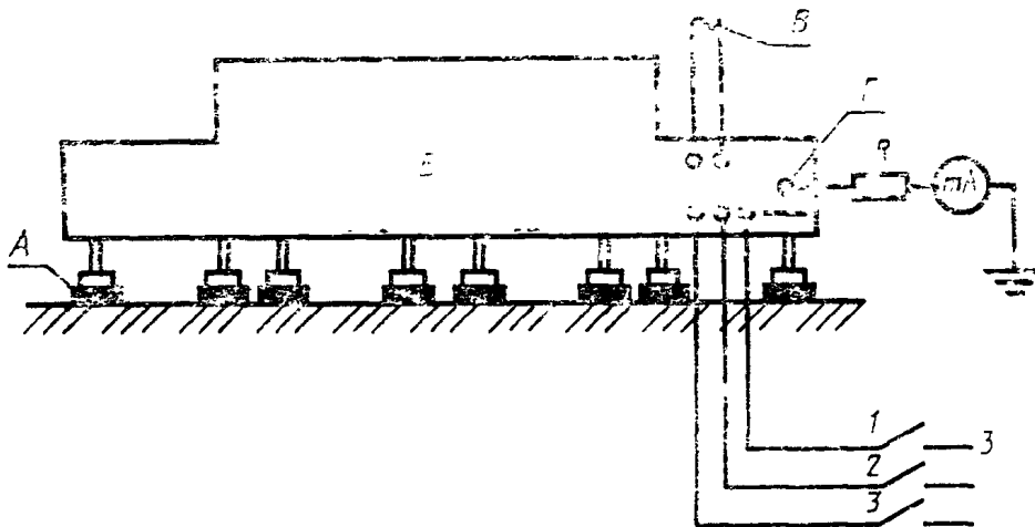
Схема измерения токов утечки посудомоечных машин
