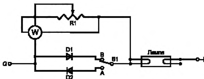
Рисунок Н.2 — Схема испытания асимметричной мощностью
