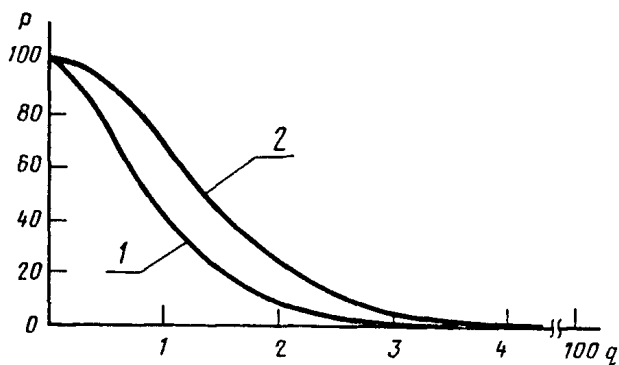
Оперативные характеристики для планов контроля значительных дефектов
