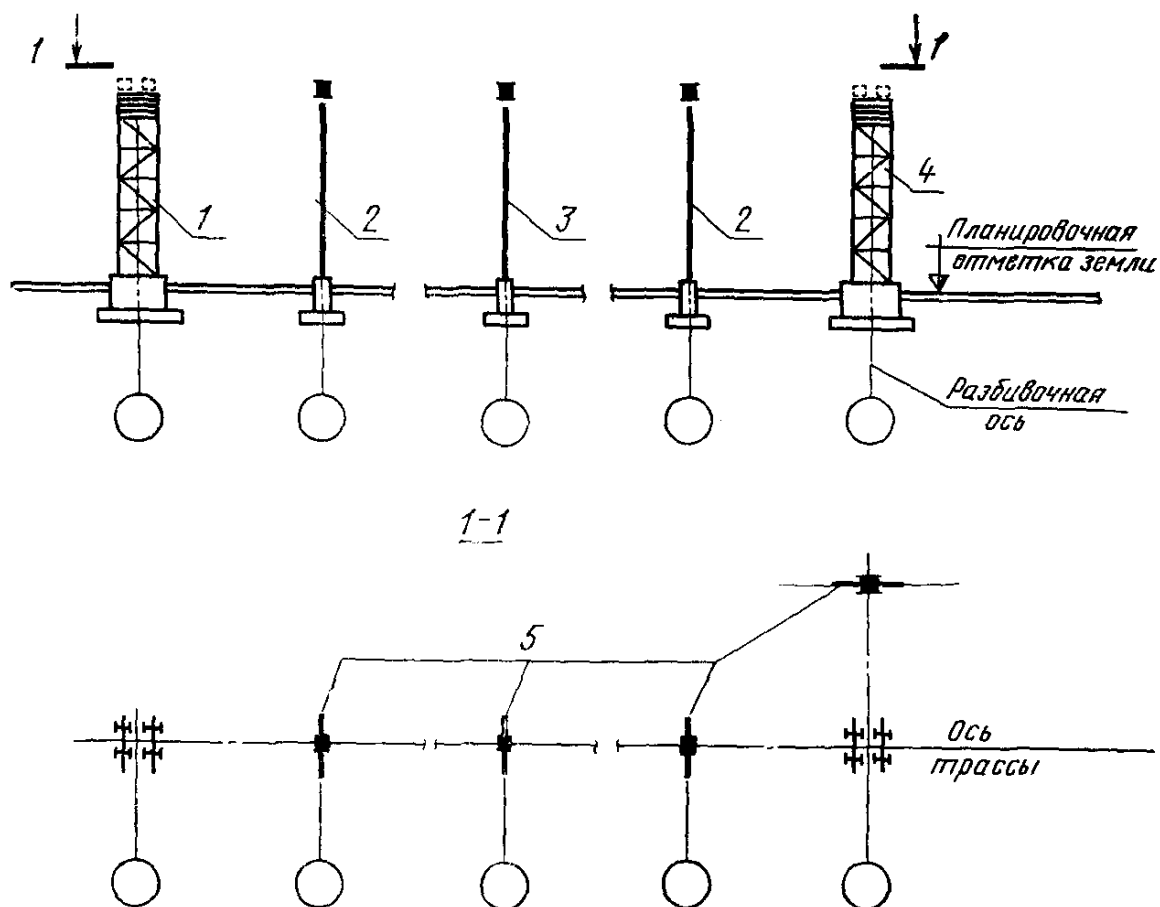
1—анкерная конечная опора; 2—промежуточная опора; 3—анкерная промежуточная опора; 4—анкерная конечная угловая опора; 5—траверса железобетонная.
