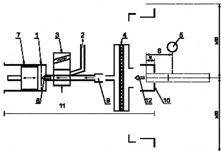
1 — положение головки поршня в начале хода; 2 — выход газовой фазы; 3 — электрочлапан; 4 — ловушка для дыма; 5 — устройство для прекращения затяжки; 6 — длина окурка; 7 — насос поршневой; 8 — перемещенный объем; 9 — отверстие; 10 — держатель сигарет; 11 — канал; 12 — объем затяжки
