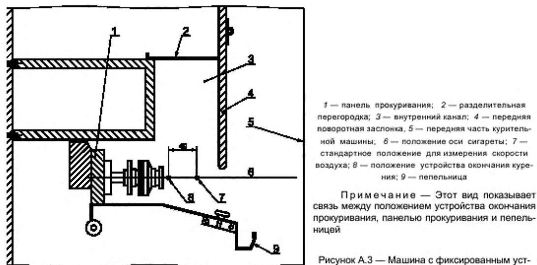
Рисунок А.3 — Машина с фиксированным уст- ройством для окончания прокуривания
