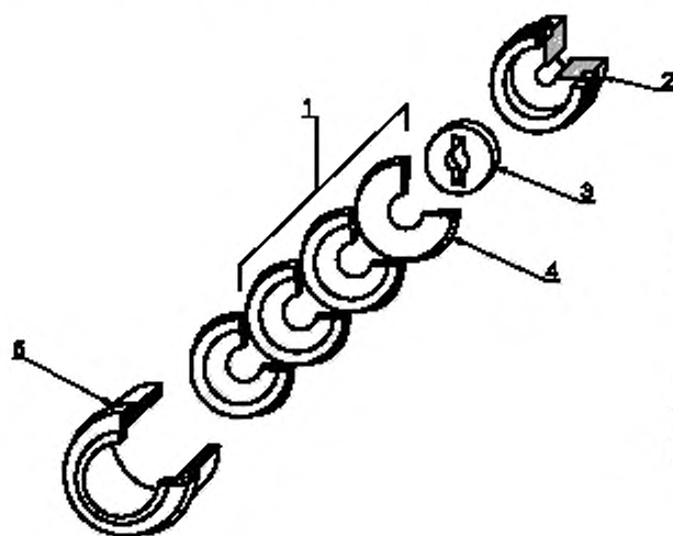
Рисунок 1 — Лабиринтное уплотнение и перфорированный диск держателя сигарет
