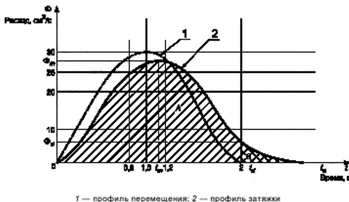
Рисунок В.1 — Схематичное изображение профиля затяжки сигареты
