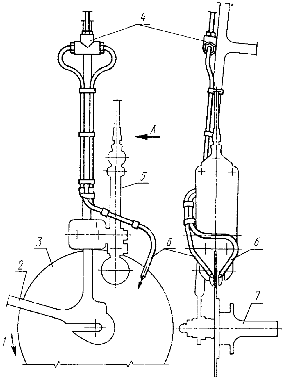
1 — направление вращения колеса; 2 — рама велосипеда; 3 — тормозной диск; 4 — задний тройник; 5 — зажим дискового тормоза; 6 — патрубок для воды; 7 — задняя втулка
