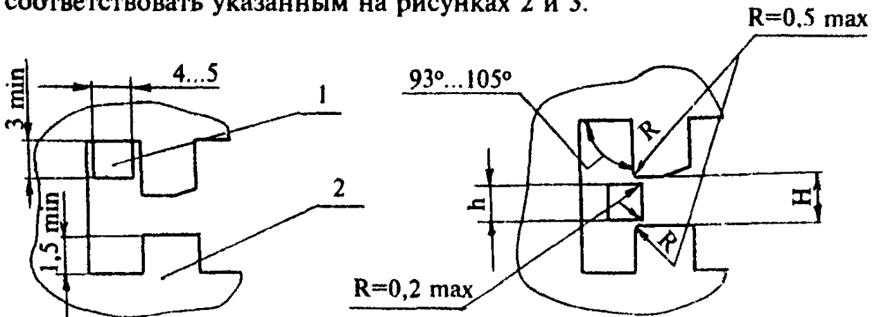
1 — стойка хвостовика; 2 — сувальда
