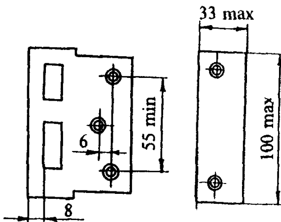
Запорная планка
