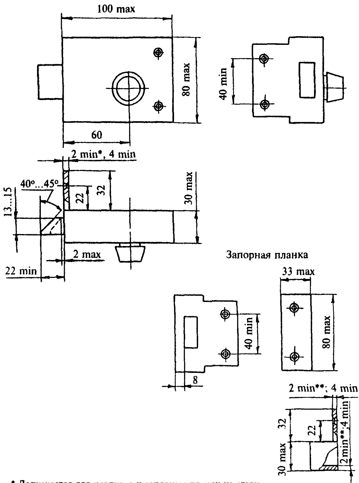
Рисунок А.7 — Замок накладной, тип 3Н2
