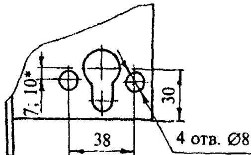
Рисунок А.1 — Замки врезные, типы ЗВ1 и ЗВ8
