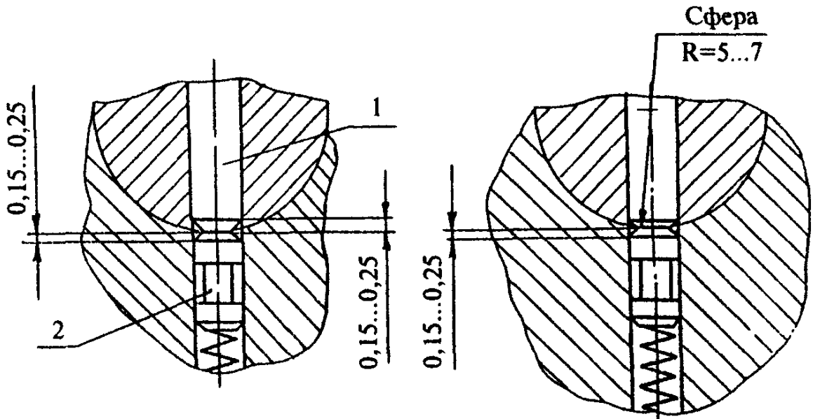
1 — штифт цилиндра; 2 — штифт корпуса
