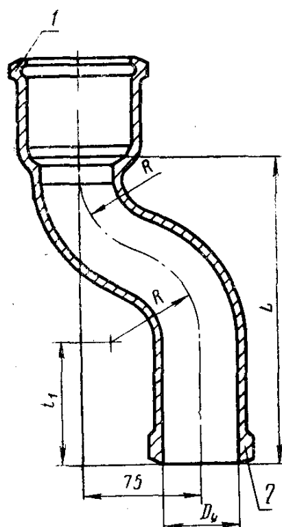
1 — раструб типа I по ГОСТ 6942.2—80; 2 — хвостовик по ГОСТ 6942.2—80
