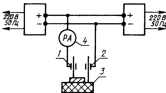
1, 2 — цанговый зажим; 3 — платиновые сетчатые электроды (комплект); 4 — амперметр
