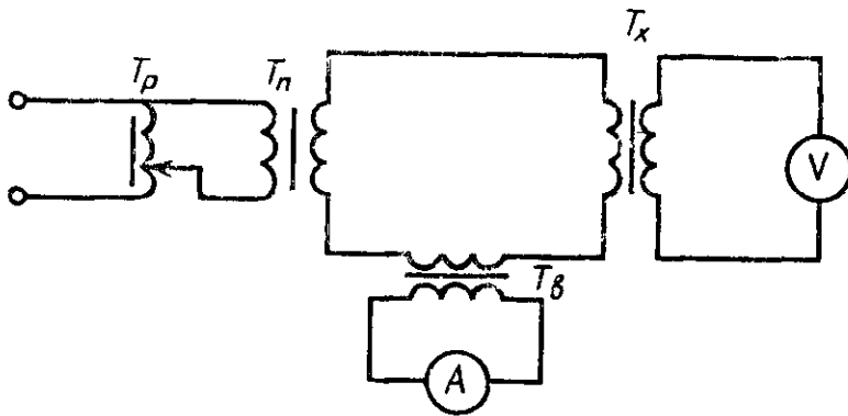
Схема размагничивания трансформатора тока
