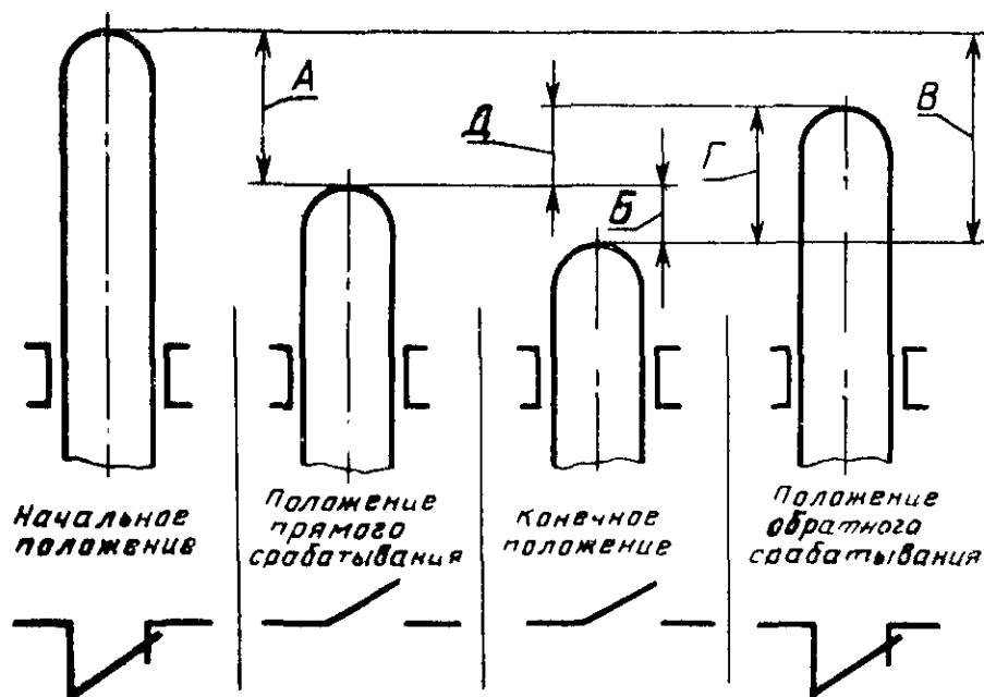
Схема положения подвижных частей выключателя
