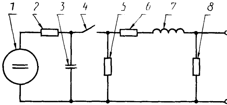
Упрощенная схема ИГ МИП
