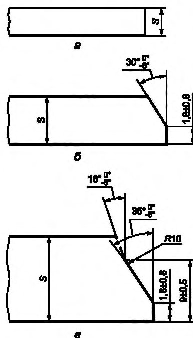
Рисунок 1 — Форма и размеры разделки торцов труб
