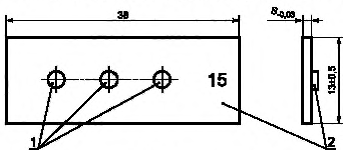
1 — отверстие \varnothing 1,6 мм; 2 — шифр пенетрометра
