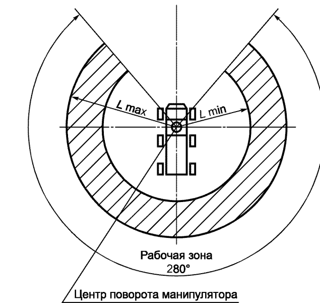
Рисунок Б.4 — Обрезка сучьев машинная
