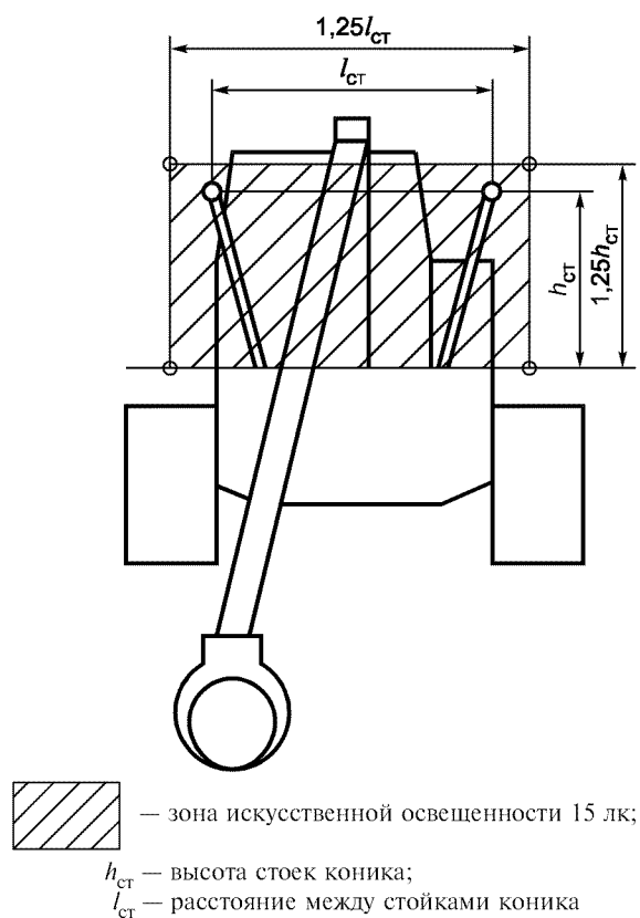
Рисунок Б.2 — Трелевка леса бесчокерная
