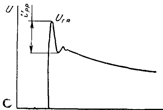
Рис. 6 Форма импульса
