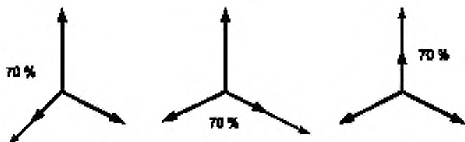
а) Испытание «фаза — нейтраль»
