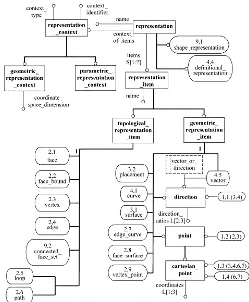
Рисунок D.1 — ПИК alic_manifold_subsurface в формате EXPRESS-G (диаграмма 1 из 9)
