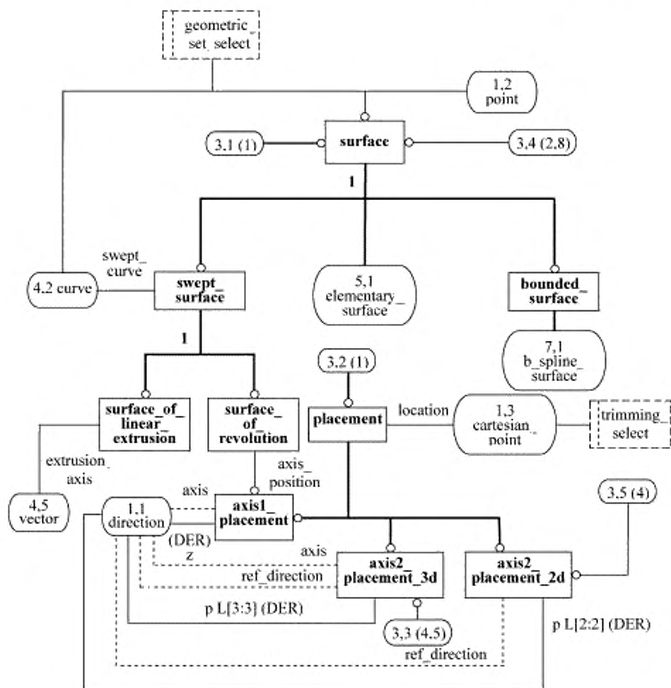
Рисунок D.3 — ПИК alc_manifold_subsurface в формате EXPRESS-G (диаграмма 3 из 9)
