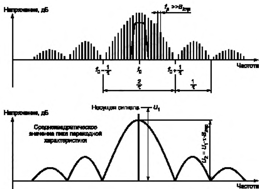
Рисунок Д.6 — Фильтрация в случае, если значения B_{\text{имп}} намного больше частоты повторения импульсов
