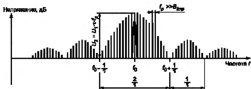
Рисунок Д.5 — Фильтрация в случае, если значение B_{имр} намного меньше частоты повторения импульсов
