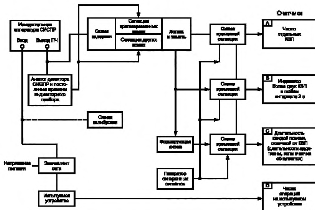
Рисунок 6 — Пример блок-схемы анализатора кратковременных ИРП
