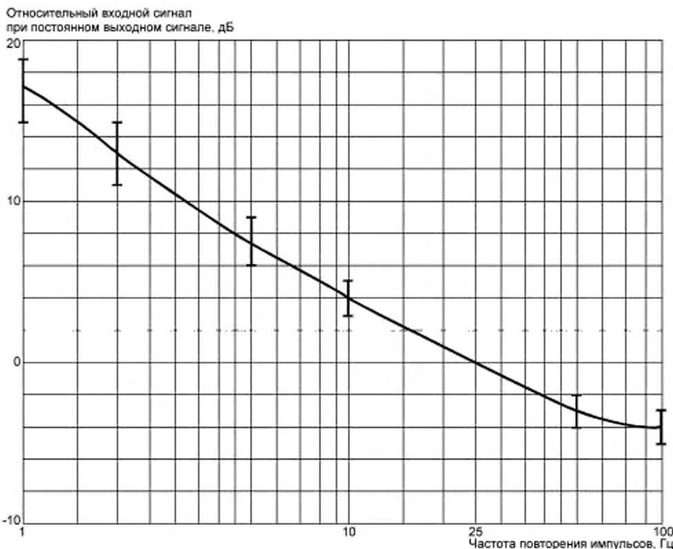
Рисунок 1 — Графики импульсных характеристик, лист 1
