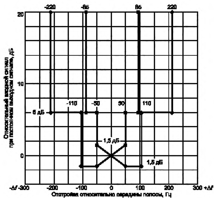
Рисунок 2 — Нормы частотной избирательности ИП, лист 1
