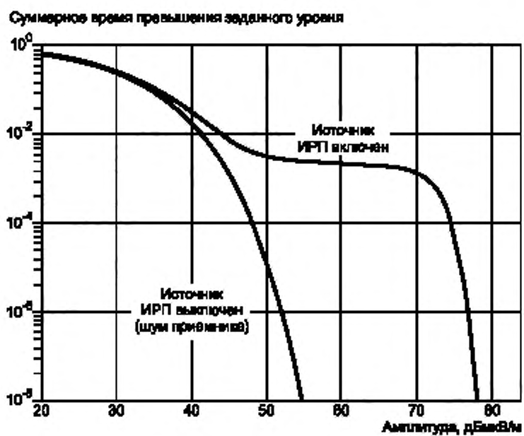
Рисунок Ж.3 — Пример функции распределения амплитуд ИРП
