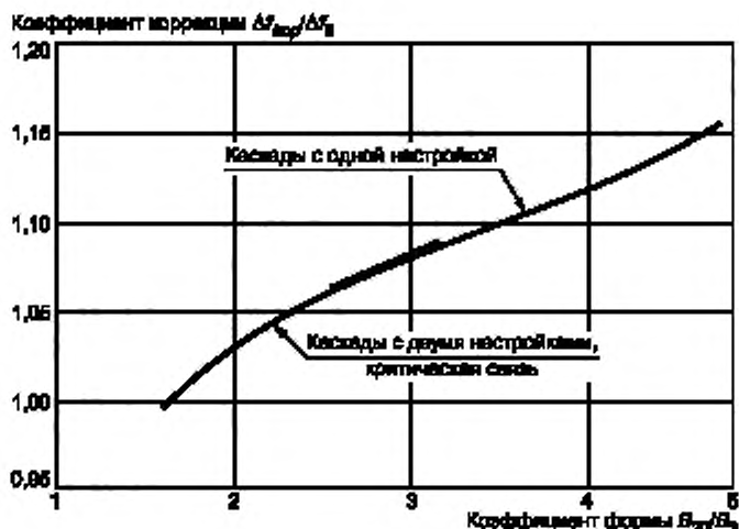
Рисунок Д.1 — Коэффициент коррекции для оценки отношения B_{имп}/B_b для других типов настраиваемых схем
