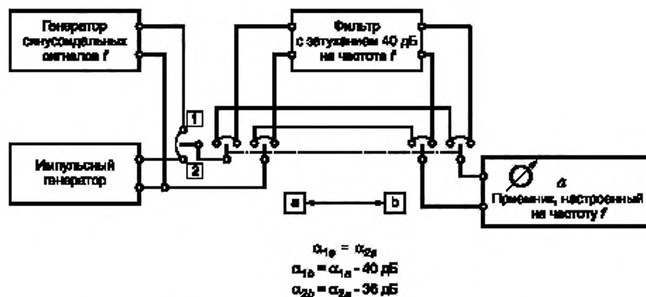
Рисунок 3 — Схема измерения ослабления продуктов интермодуляции
