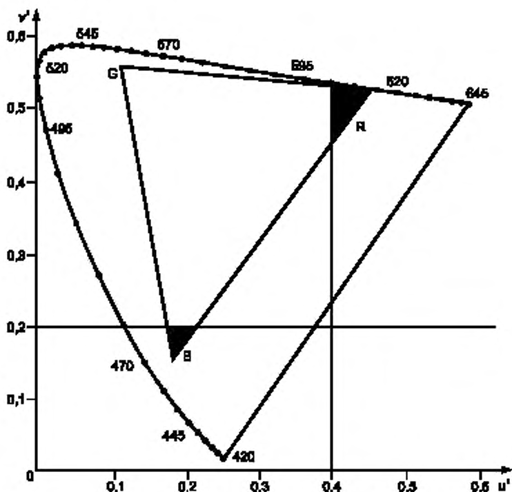
Рисунок 5 — Спектральное ограничение цветов
