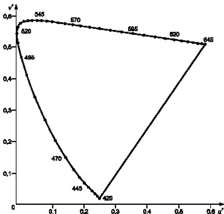
Рисунок 1 — Равноконтрастный цветовой график МКО 1976 г.
