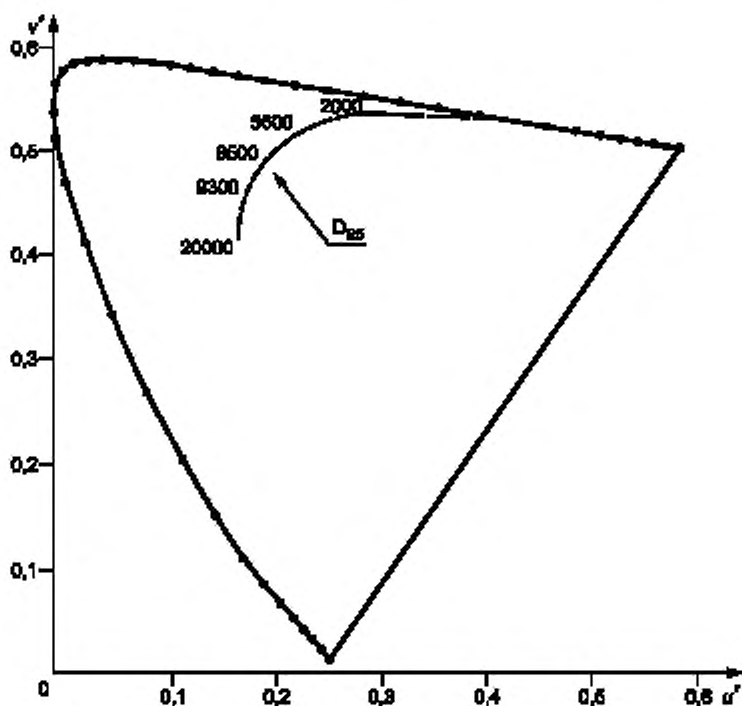
Рисунок 2 — Положение иллиминанта МКО D 65 и цветных температур на равноконтрастном цветовом графике МКО 1976 г.
