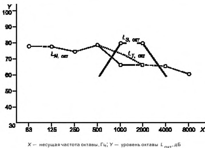
Рисунок D.1 — График анализа окружающего шума в полосе октавы, эффективного маскирующего предела и сигнала опасности в течение периода «вкл.»
