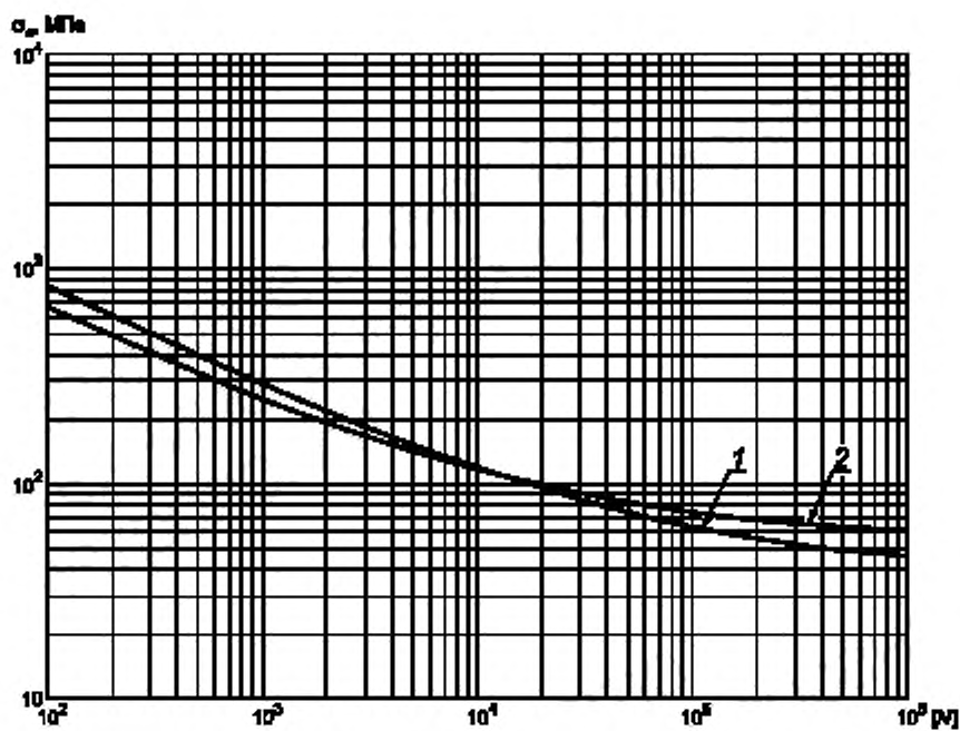
Рисунок 7 — Расчетная кривая усталости для сплавов меди
