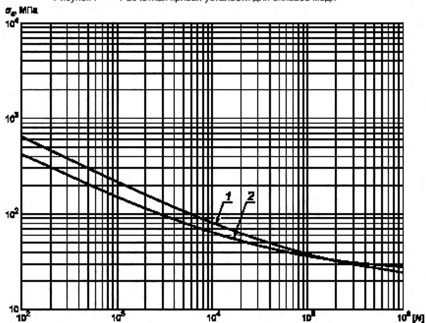
Рисунок 7 — Расчетная кривая усталости для сплавов меди
