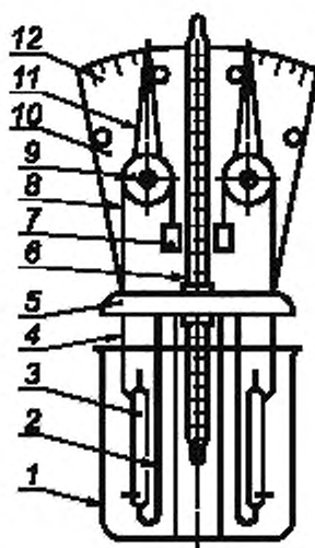
1 — стакан; 2 — неподвижный крючок; 3 — образец кожной ткани; 4 — подвижной крючок; 5 — металлическая пластина; 6 — термометр; 7 — груз; 8 — прочная нить; 9 — шкив; 10 — вертикальная стойка; 11 — подвижная стрелка; 12 — шкала
