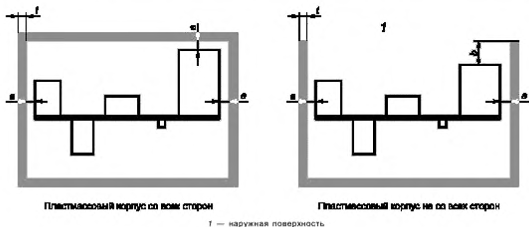
Рисунок 3 — Расстояния между стенкой или открытой поверхностью компаунда и элементами или проводниками
