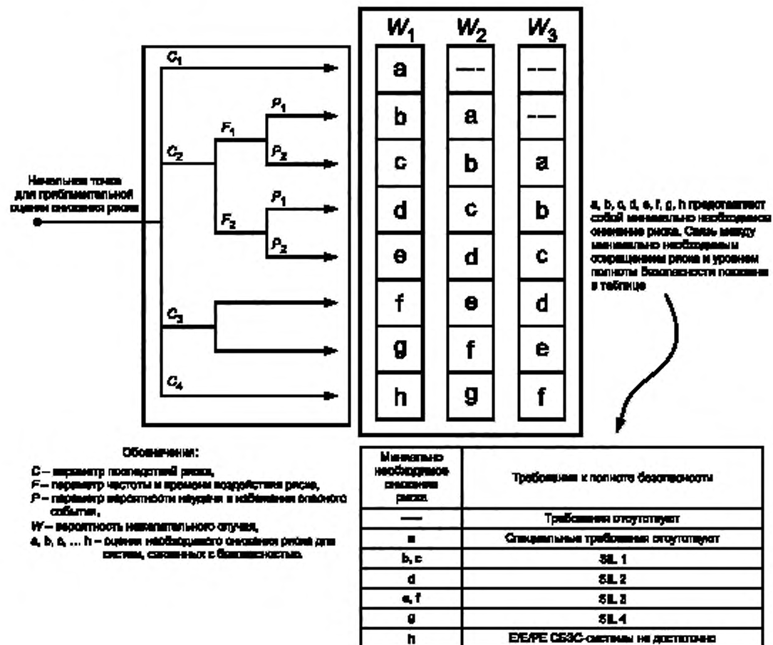
Рисунок Ж.2 — Пример реализации графа риска
