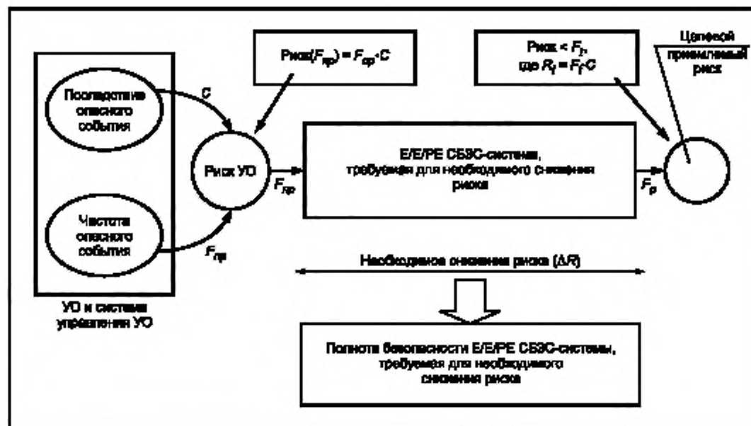
Рисунок E.4 — Схема расчета целевой полноты безопасности одиночной E/E/PE CBZC-системы
