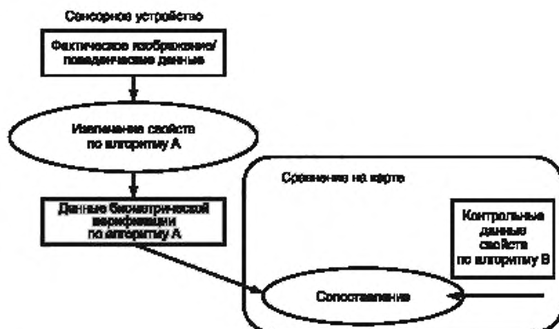
Рисунок А.3 — Использование данных свойств в сценарии сравнения на карте
