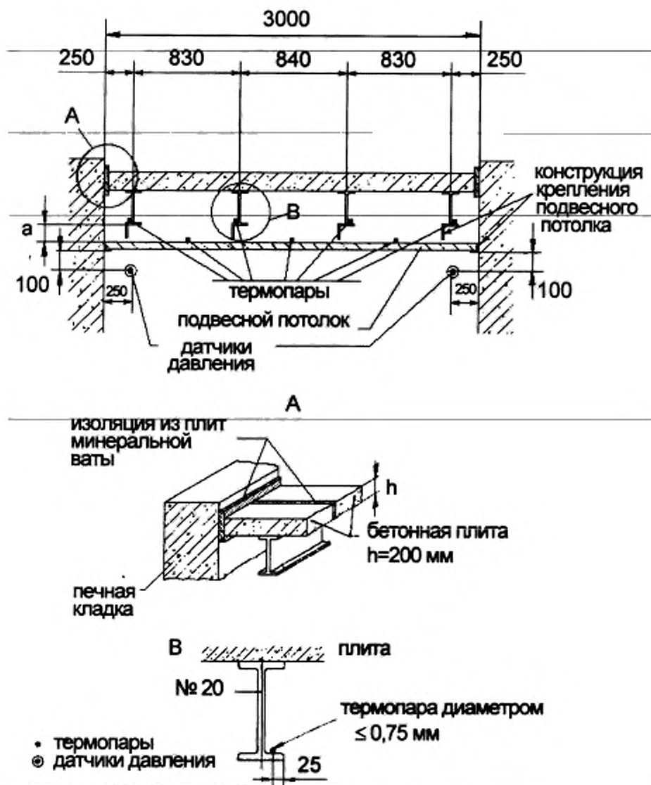
Рисунок А.1 — Схема испытательного блока
