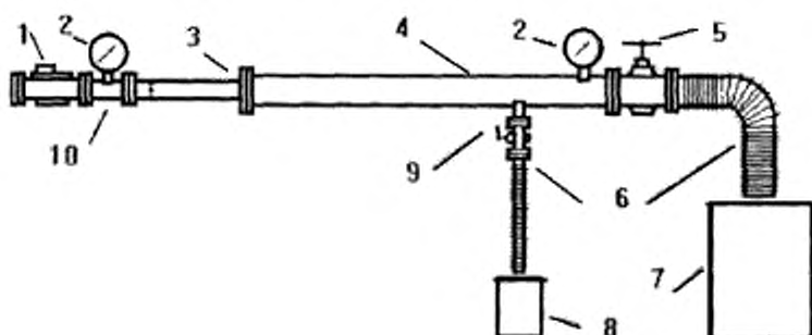
1 — расходомер; 2 — манометры; 3 — пеногенератор; 4 — основной трубопровод; 5 — задвижка; 6 — эластичные рукава; 7, 8 — емкости на 2000 и 10 л; 9 — шаровой кран; 10 — дополнительный трубопровод
