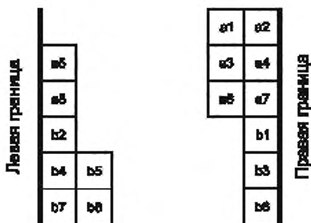
Рисунок F.1 — Правый и левый знаки символа
