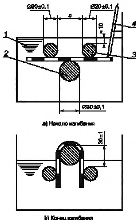
Рисунок 1 — Конструкция и принцип действия изгибающего приспособления
